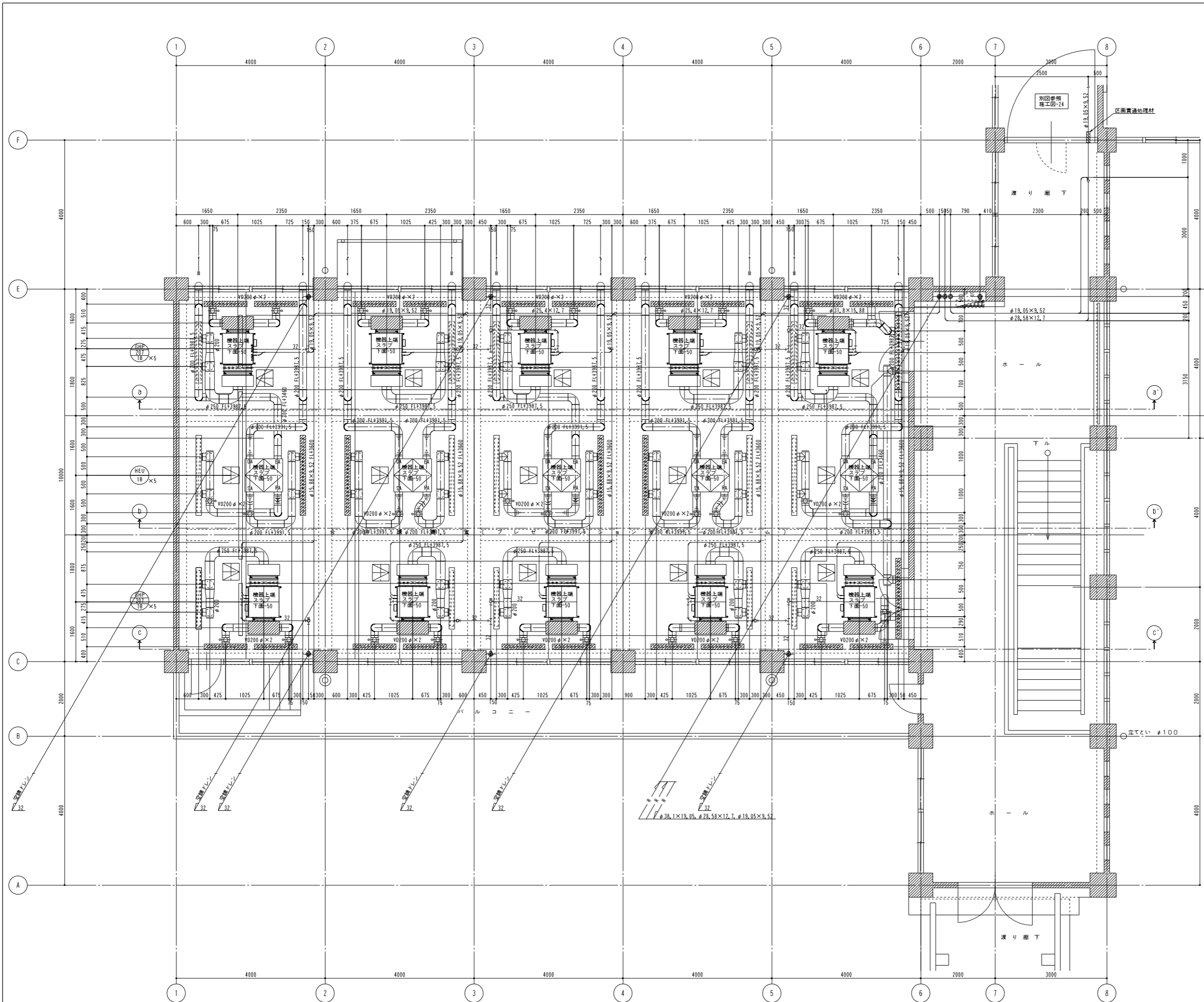
ボックス詳細図 1/30 [ハッチング部はGW25t内張]
