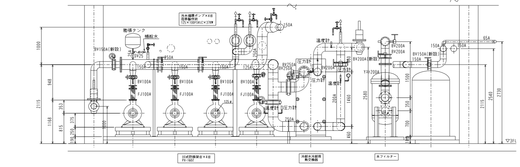
断面 1/30
